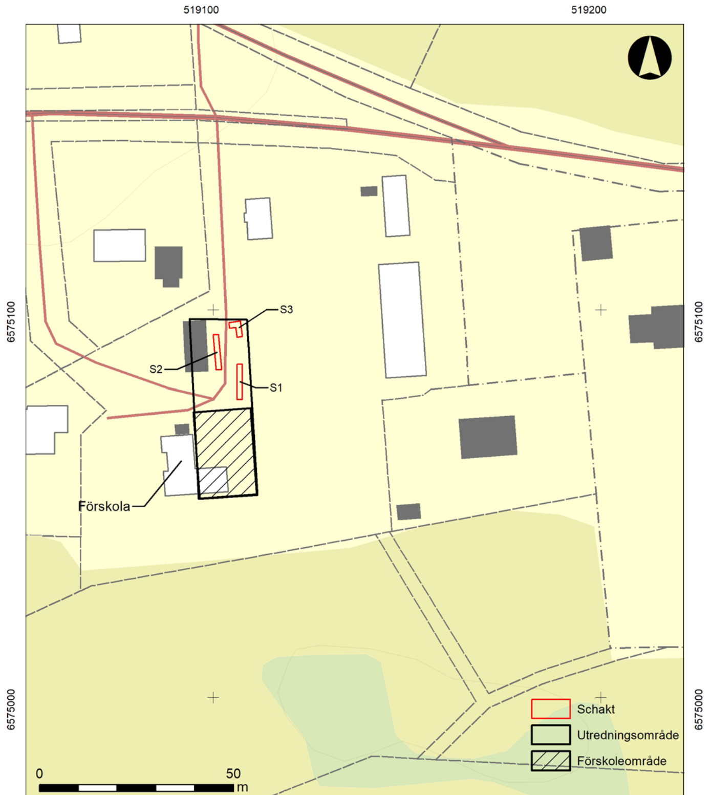
Figur 3. Schaktplan. Skala 1:1 000.
