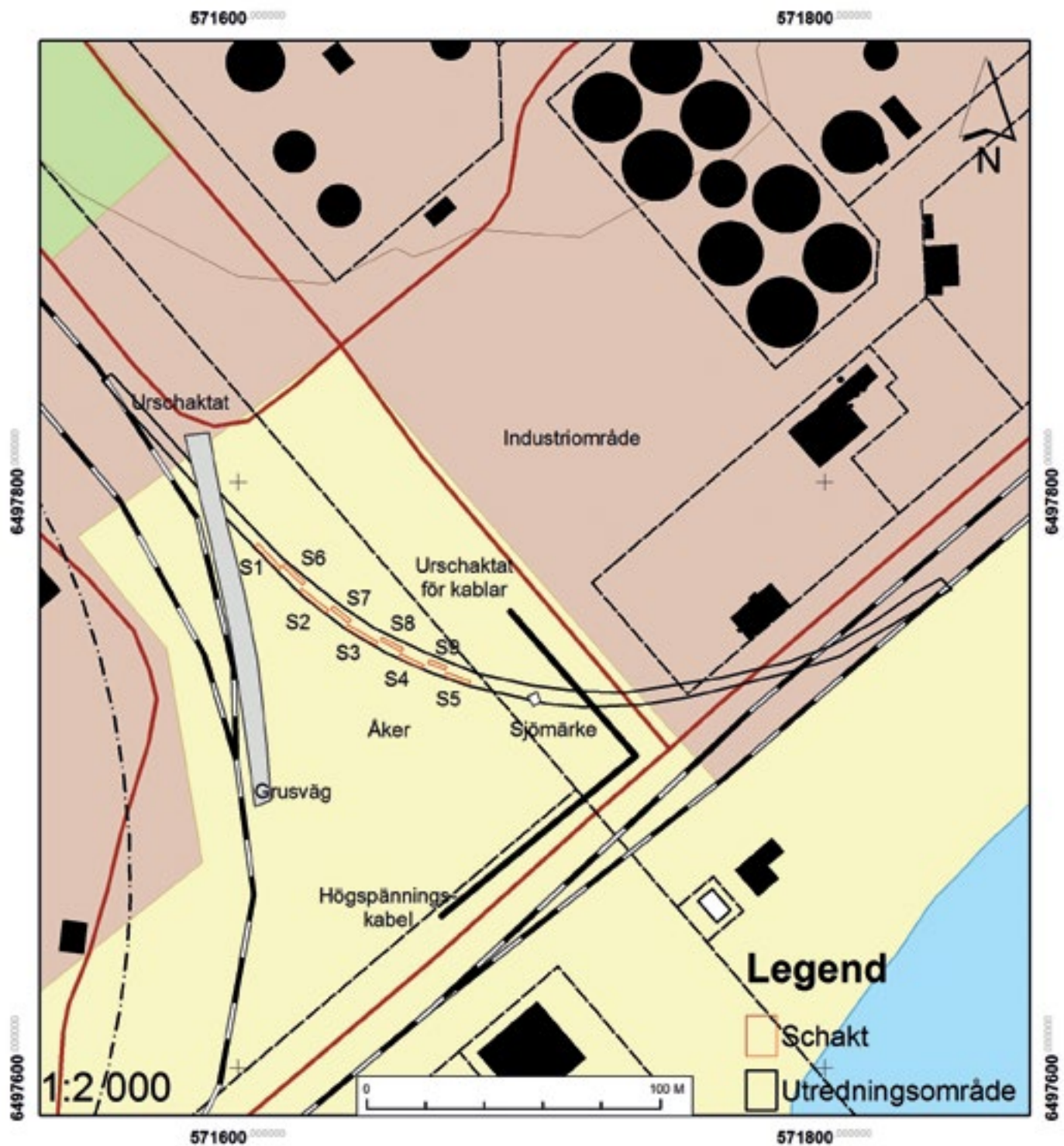
Figur 3. Schaktplan över utredningsområdet samt förklaringar över markanvändandet.
