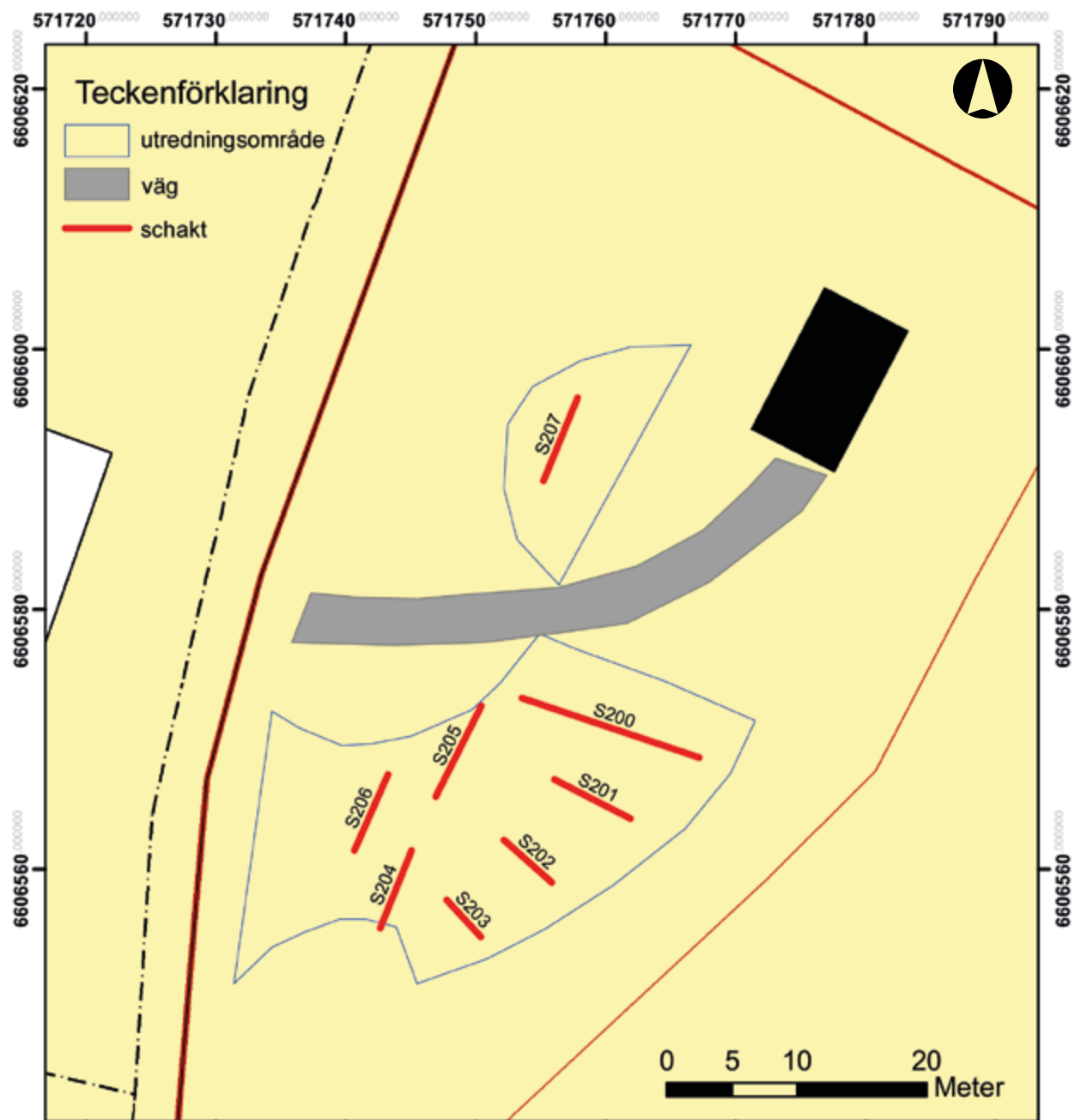
Figur 3. Plan över utredningsschakten. Skala 1:500.
