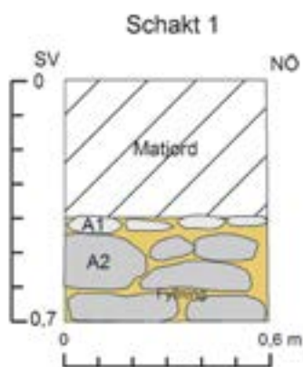
Figur 3. Profil över schakt 1. Skala 1:20.
