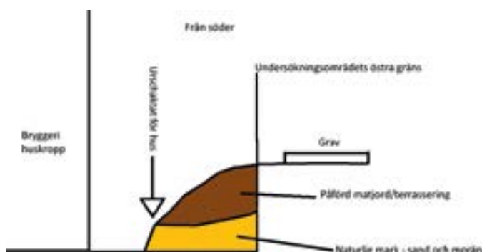
Figur 5. Sektion (V-Ö) genom undersökningsområdet sedd från söder. Skala 1:100.
